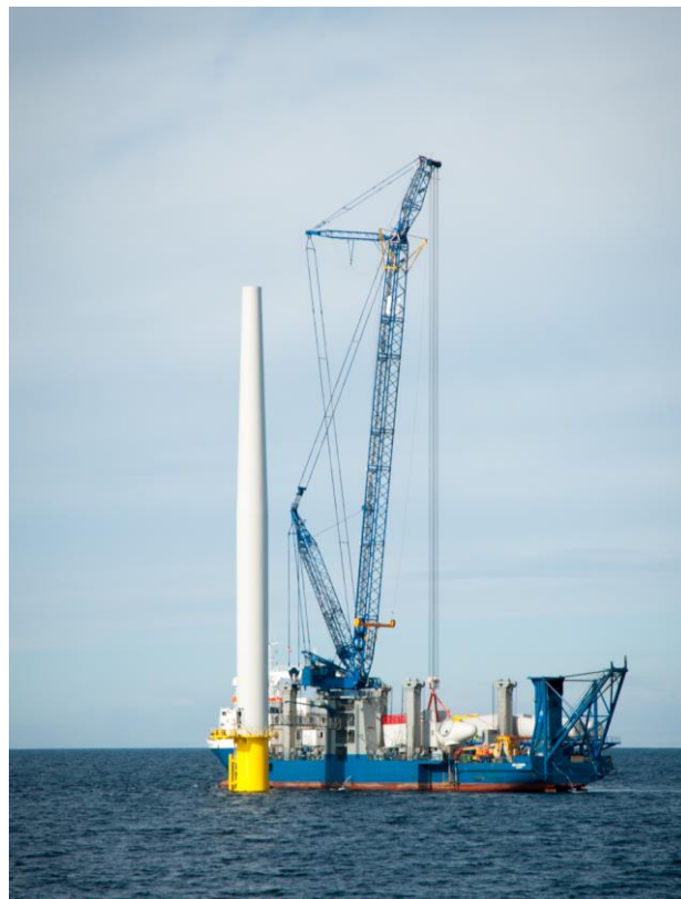
Figur 4-1 Installation av turbin med semi-jack-up fartyg vid Anholt. (Foto: Ramboll)
