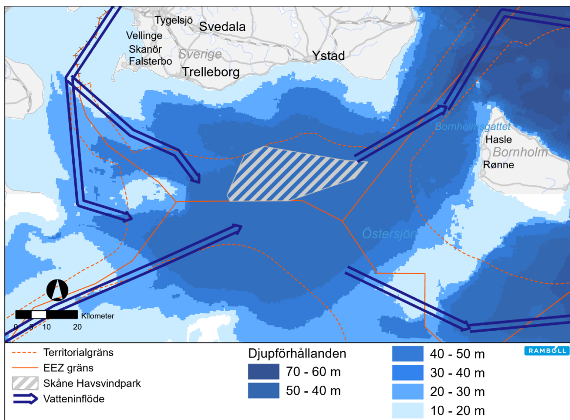
Figur 7-6 Batymetri (HELCOM, 2021) . Inflödesvägarna för saltvatten indikeras med blå pillar (Mohrholz, Naumann, Nausch, Krüger, & Gräwe, 2015).
