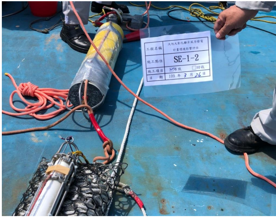
本季水下噪音儀器 SE-1-2 現場補佈放
