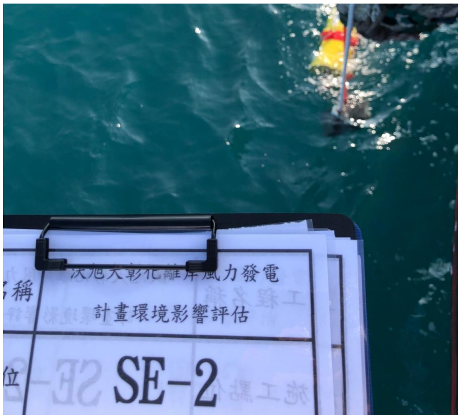
本季水下噪音儀器 SE-2 現場佈放(2/2)
