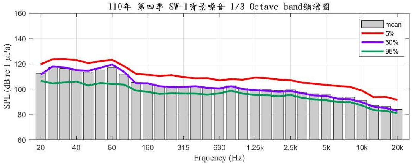
圖 2.6-11 110 年第四季 SW-1 背景噪音 1/3 Octave band 頻譜圖
