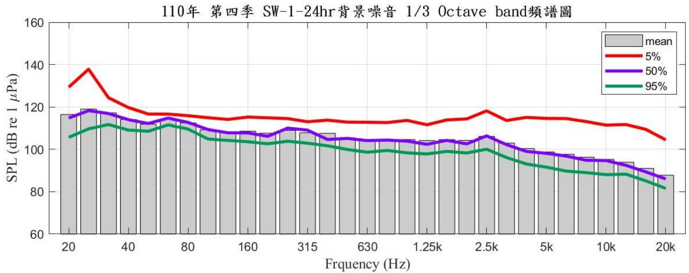
圖 2.6-12 110 年第四季 SW-1 背景噪音 1/3 Octave band 頻譜圖(補測)
