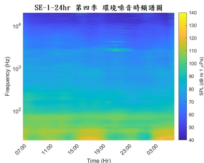
圖 2.6-6 110 年第四季 SE-1 背景噪音時頻譜圖 (補測)
